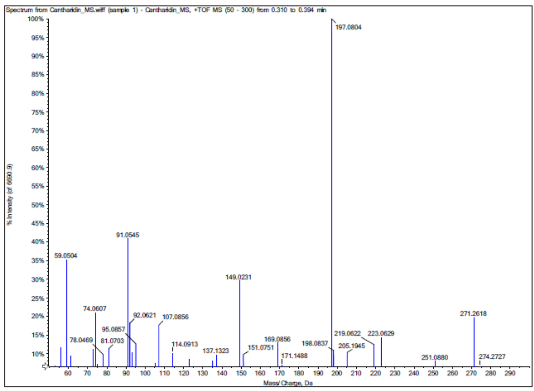
Fig4 ESIMS of C
