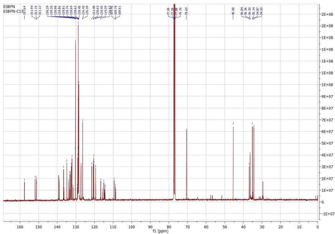
7. 4,5-bis(2-([4-(2-benzyl)phenoxy]benzyl]thio) ethoxy) phthalonitrile ( 2 ) ^{13}\text{C} -NMR Spectrum
