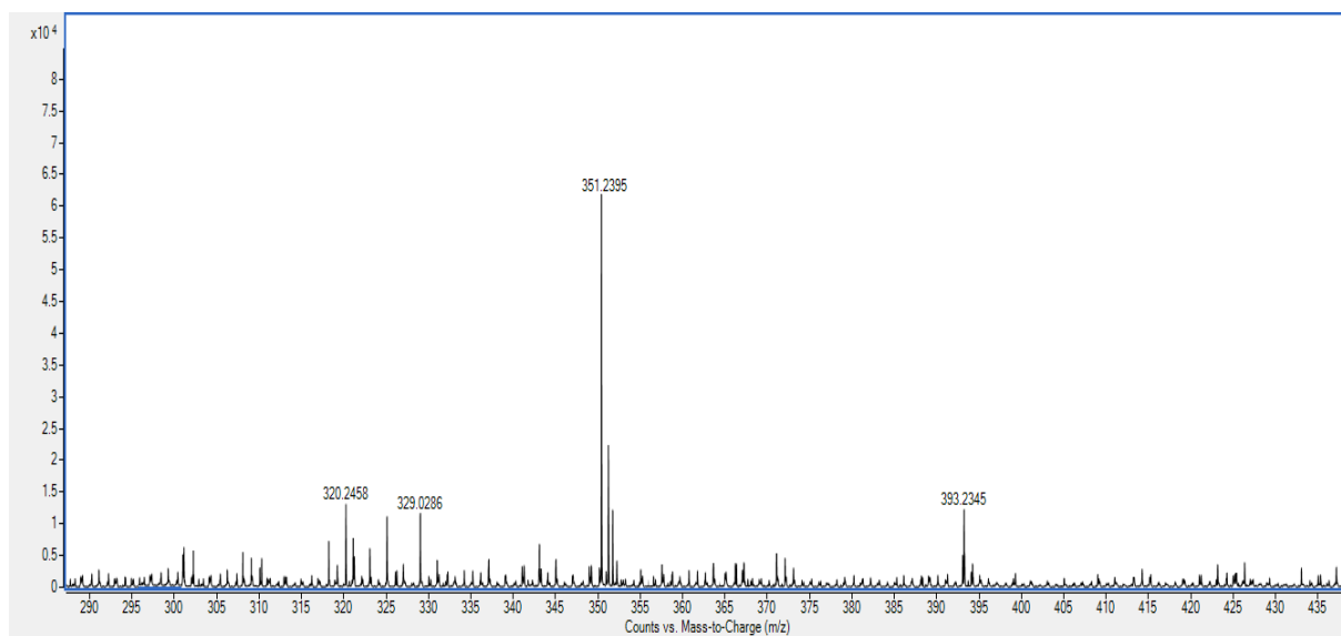
4. 2-([4-(2-benzylphenoxy)benzyl]thio)ethanol ( 1 ) Mass Spectrum
