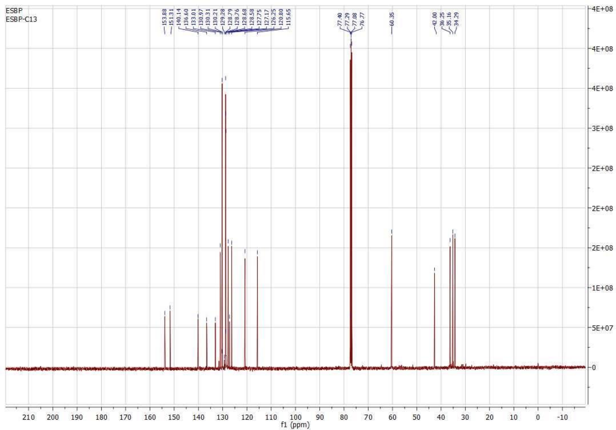
3. 2-([4-(2-benzylphenoxy)benzyl]thio)ethanol ( 1 ) ^{13}\text{C} -NMR Spectrum
