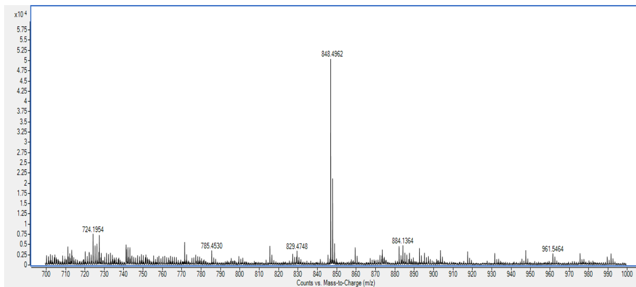
8. 4,5-bis(2-([4-(2-benzyl)phenoxy]benzyl]thio) ethoxy) phthalonitrile ( 2 ) Mass Spectrum
