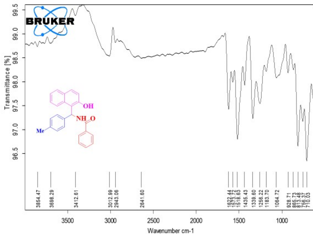
IR Spectrum of compound 4e , Table 3
